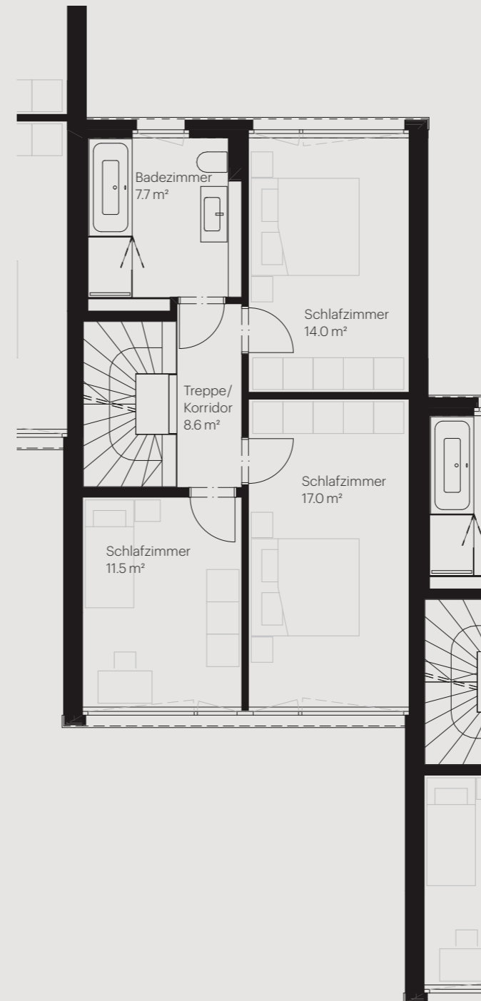
Obergeschoss
