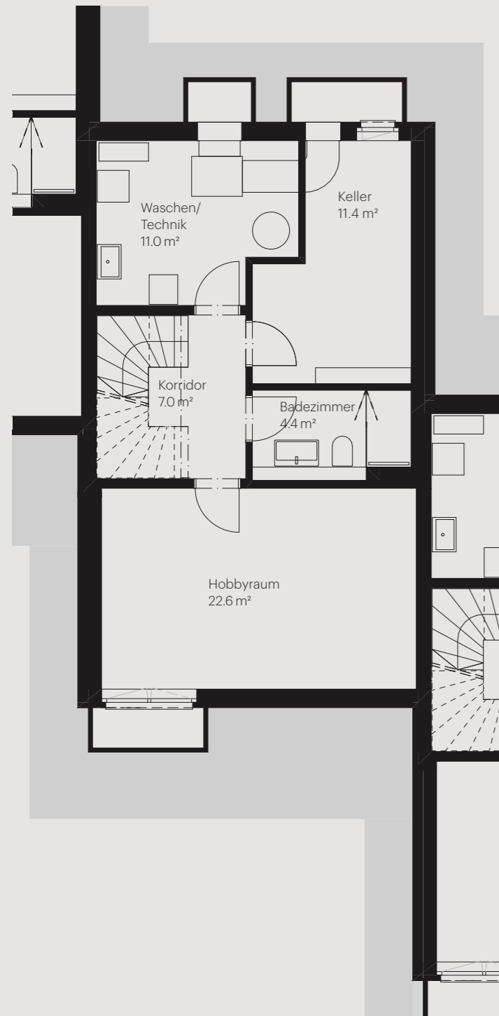
Untergeschoss
