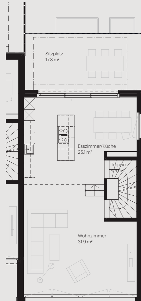
Erdgeschoss
