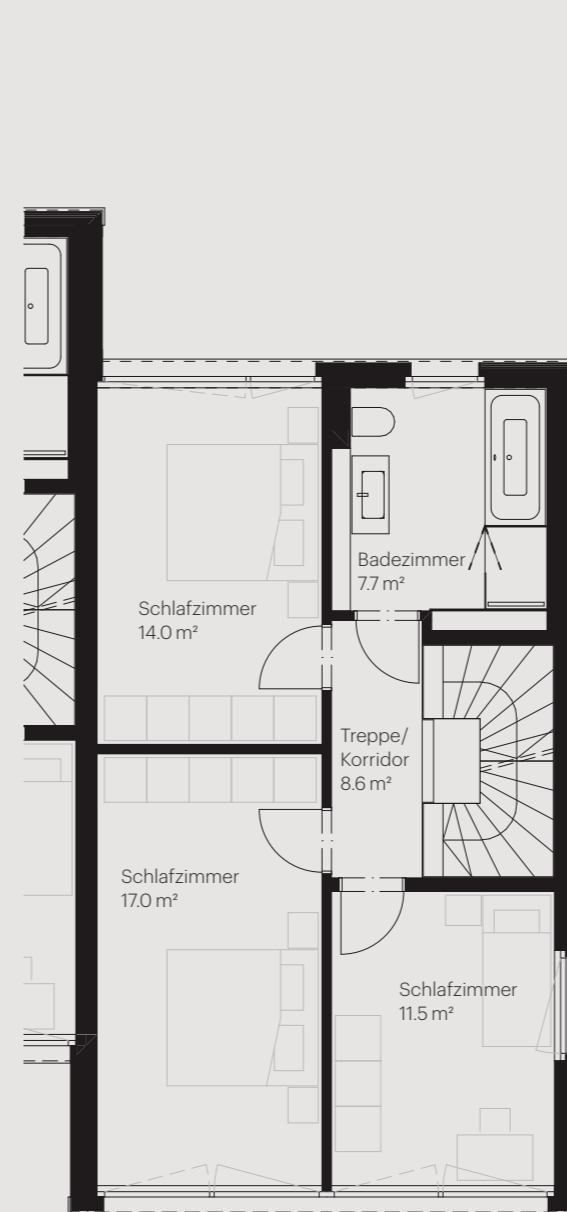
Obergeschoss
