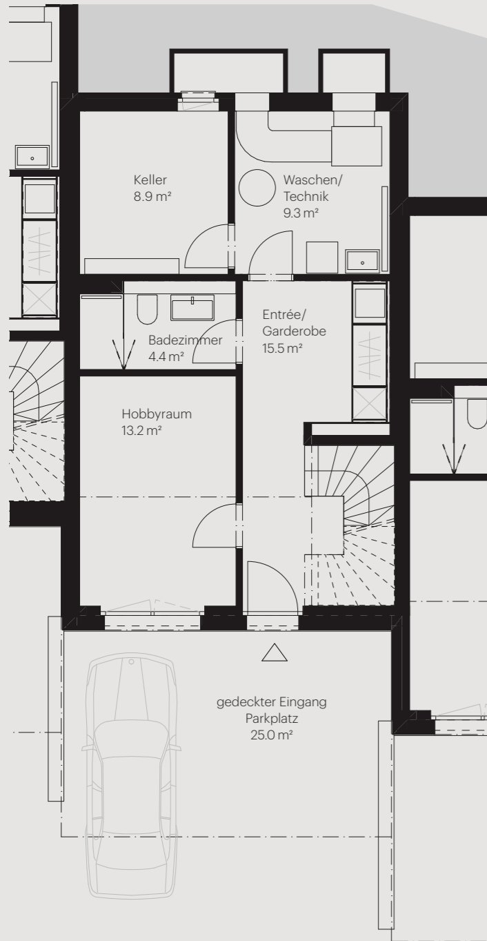
Untergeschoss
