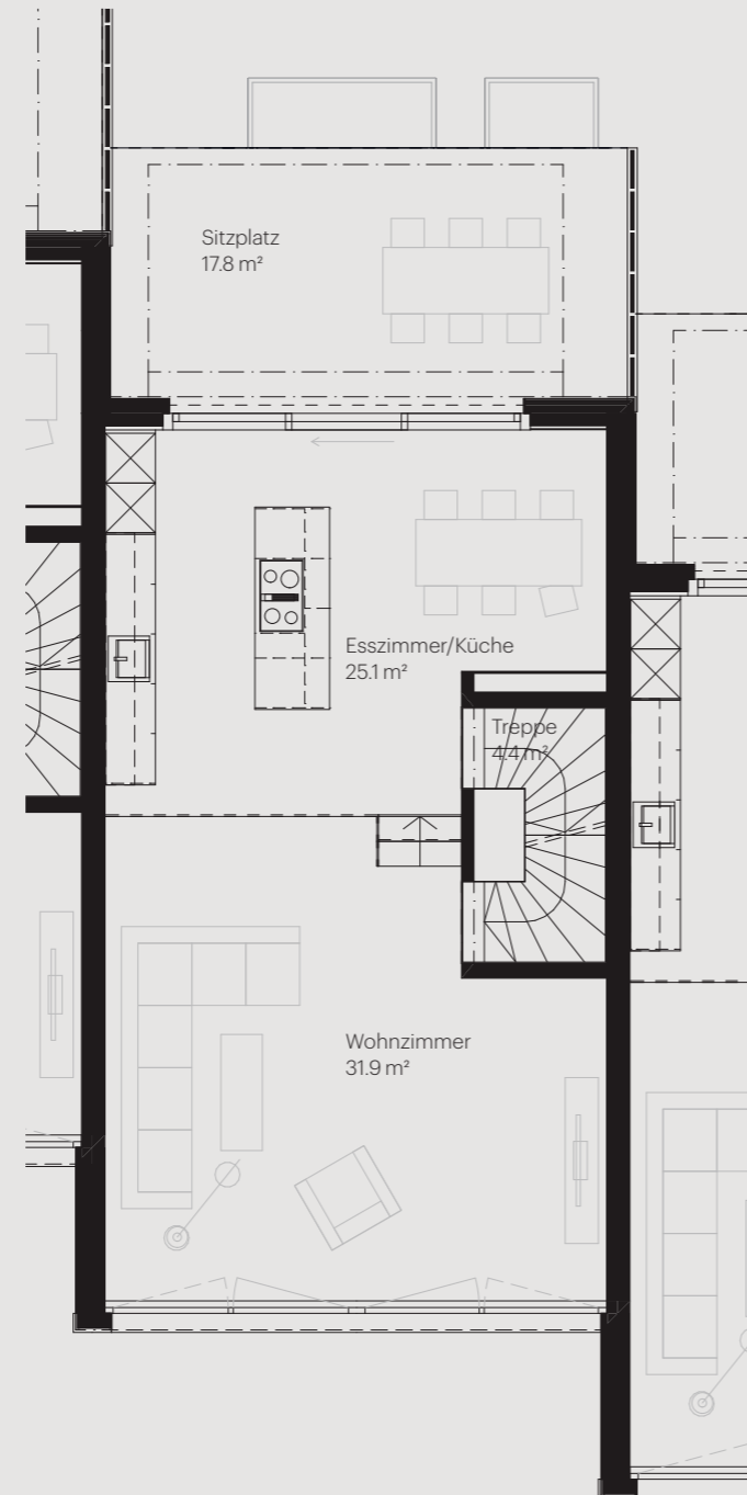
Erdgeschoss
