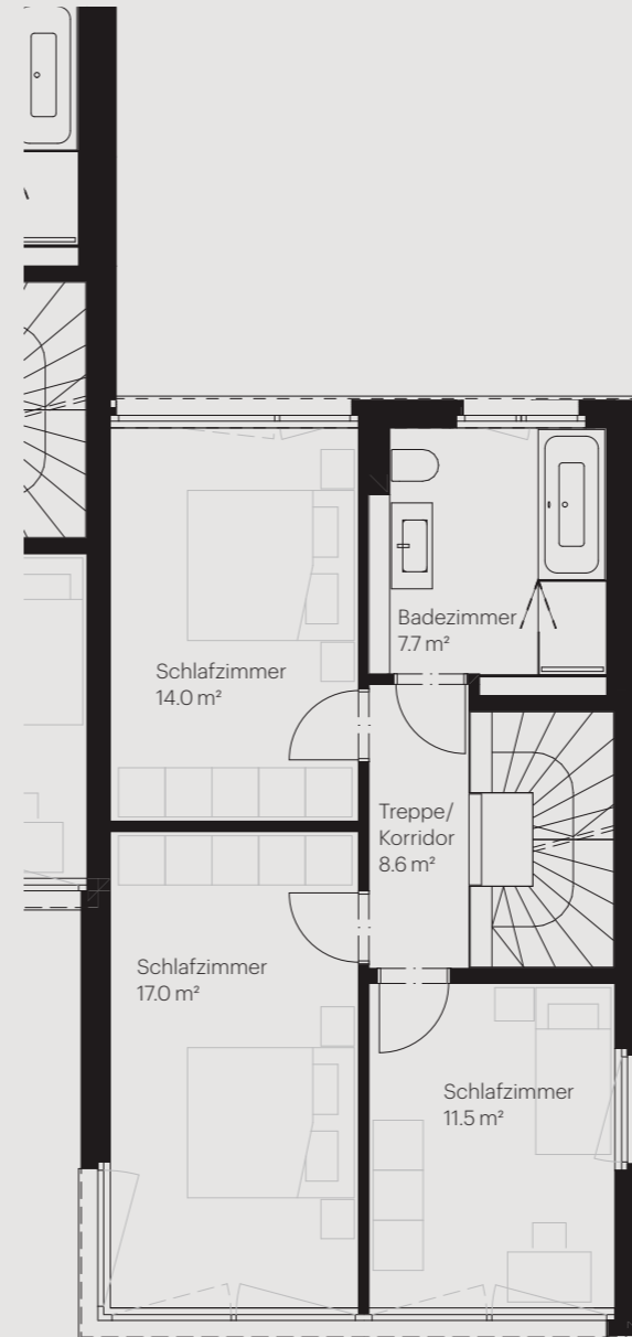
Obergeschoss
