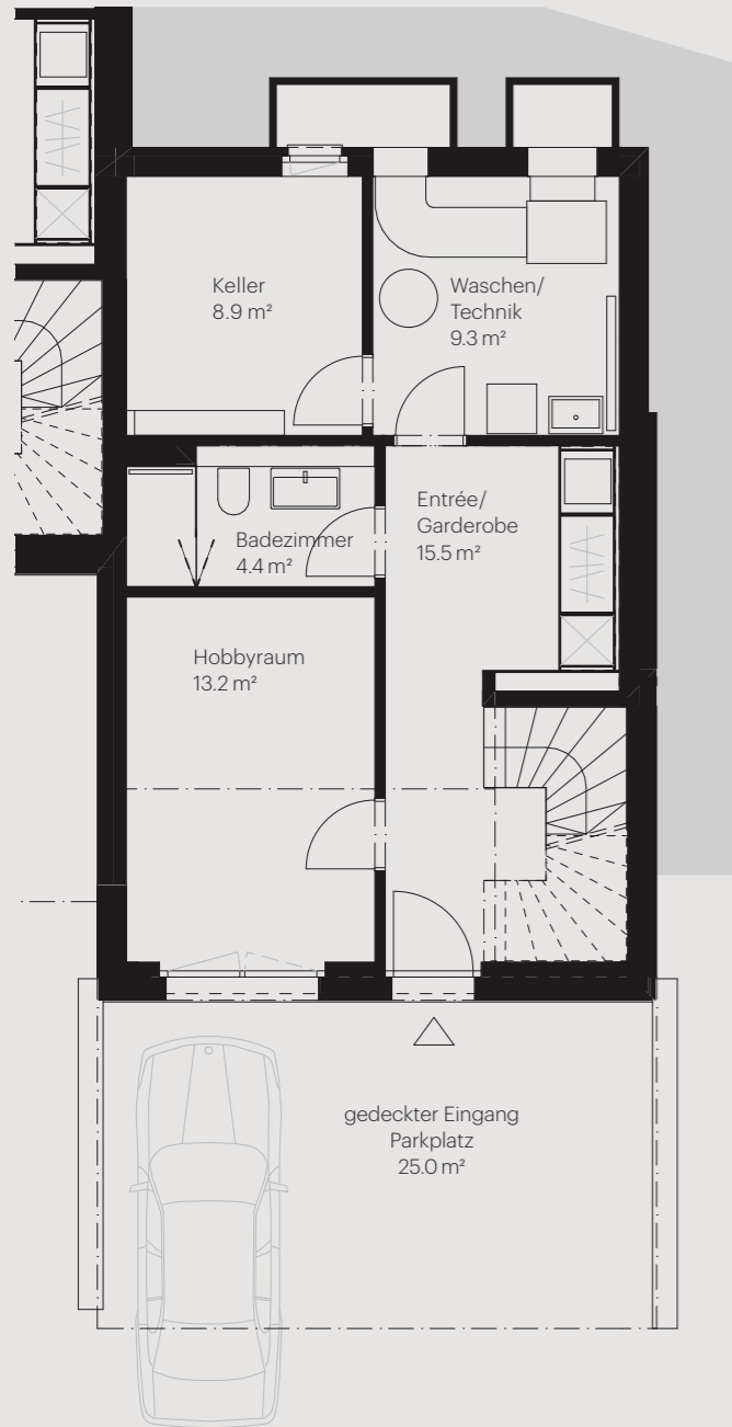
Untergeschoss
